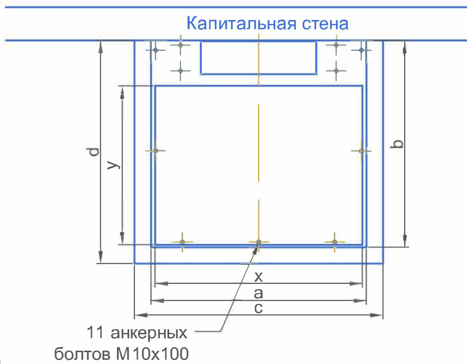
Рекомендуемые минимальные размеры фундамента
